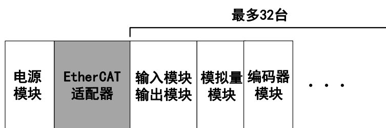
图2.3 EtherCAT总线适配器及本地扩展模块
