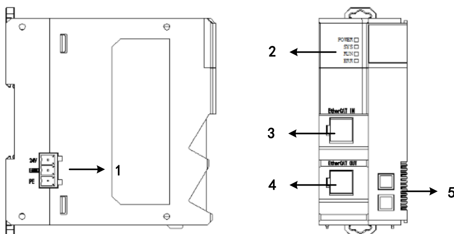
图5.14 PM32EC-A0的接口和指示灯编号
