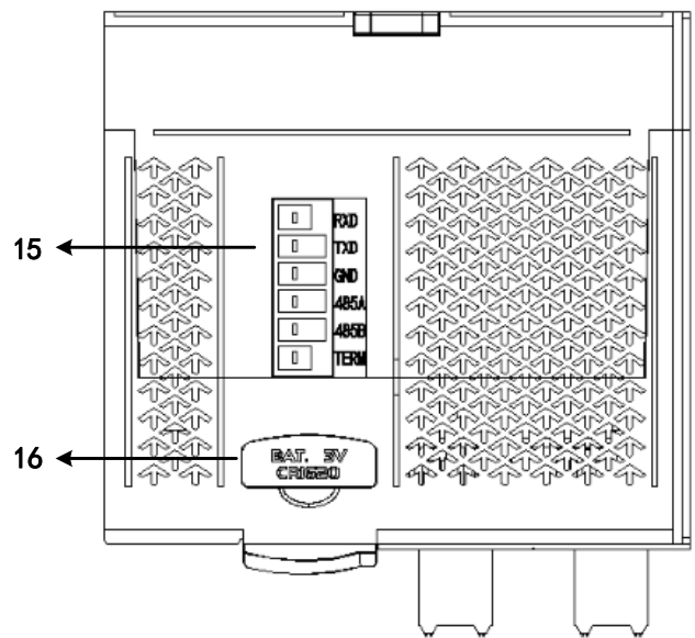
图3.5 主机俯视图各部件编号
