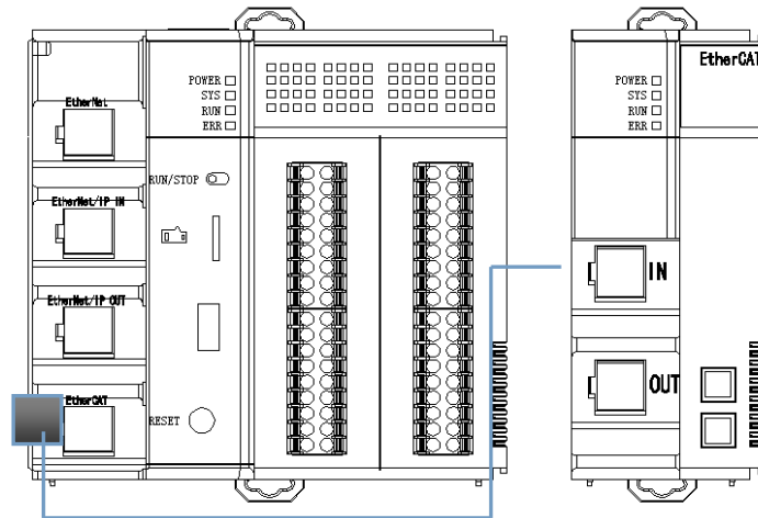
图3.14 PMC600主机的EtherCAT接口与EtherCAT通信适配器的连接
