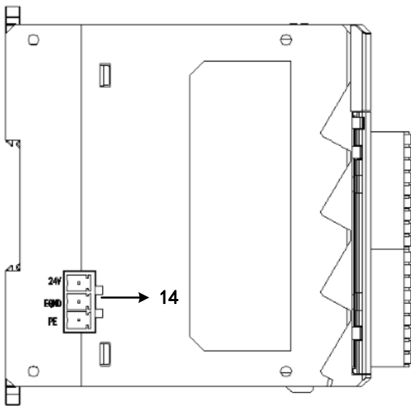
图3.4 主机左视图各部件编号
